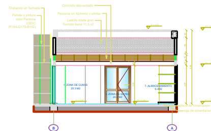
CORTE B - B ESC. 1:75
