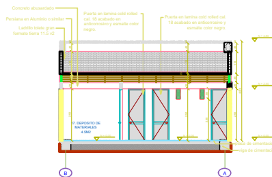
CORTE B - B ESC. 1:75
